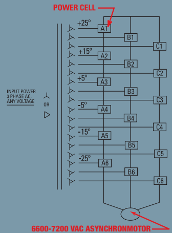
6600-7200 VAC ASYNCHRONMOTOR
